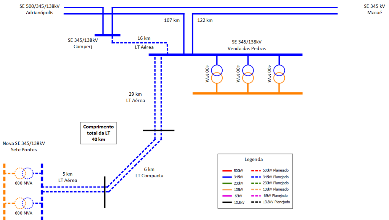
Figura 3-2 - Representação simplificada da alternativa 3A
