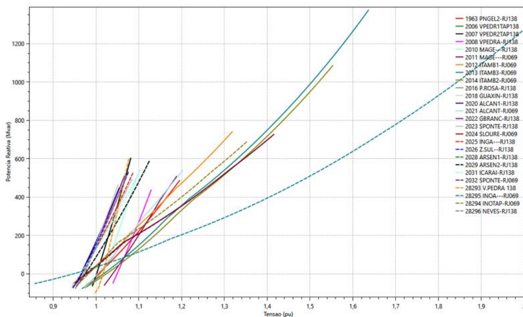
Figura 5-1 - Curva QxV - Sistema Niterói, Carga Pesada 2024
