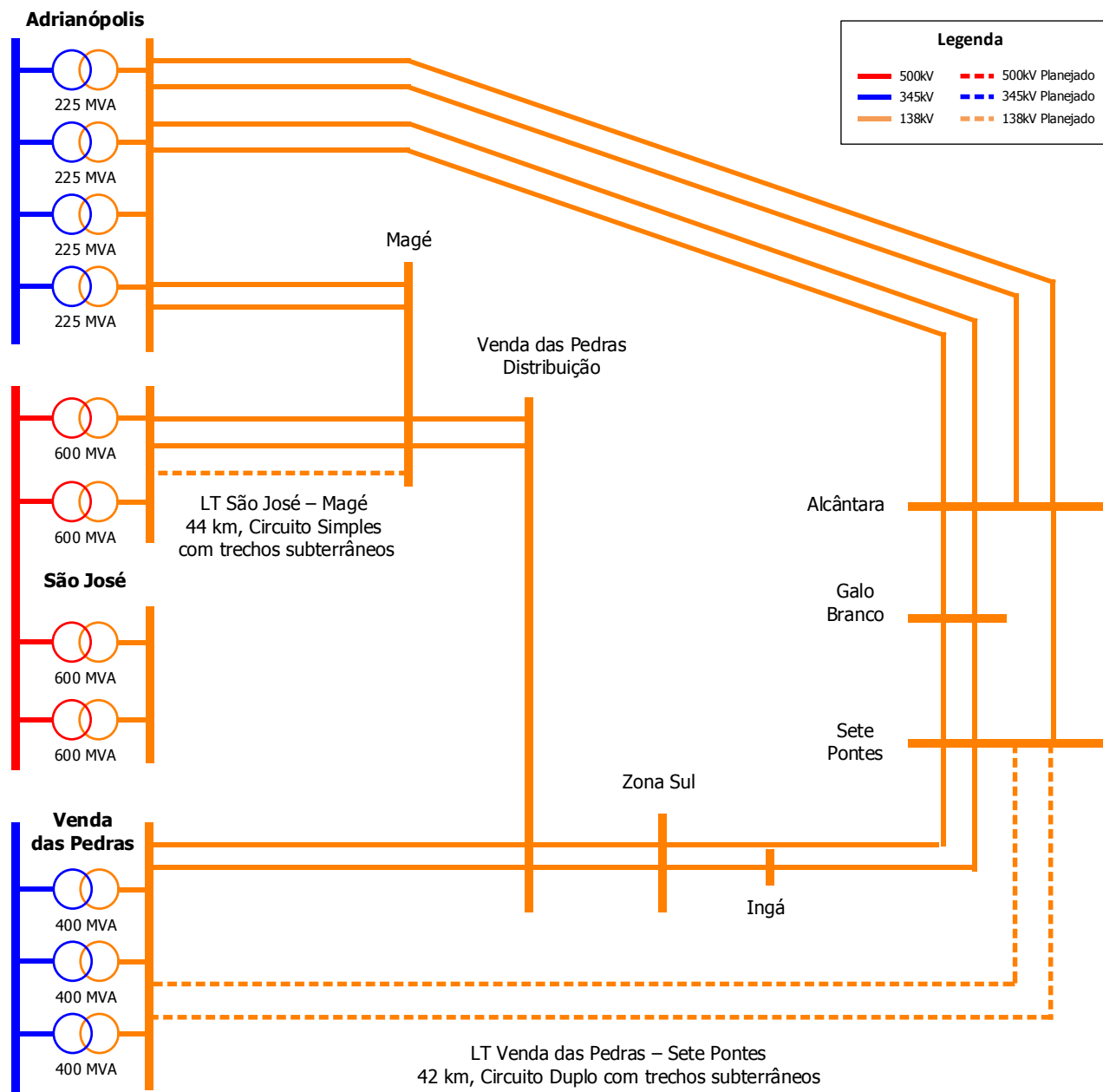
Figura 6-7 - Diagrama simplificado das principais obras da Alternativa 4
