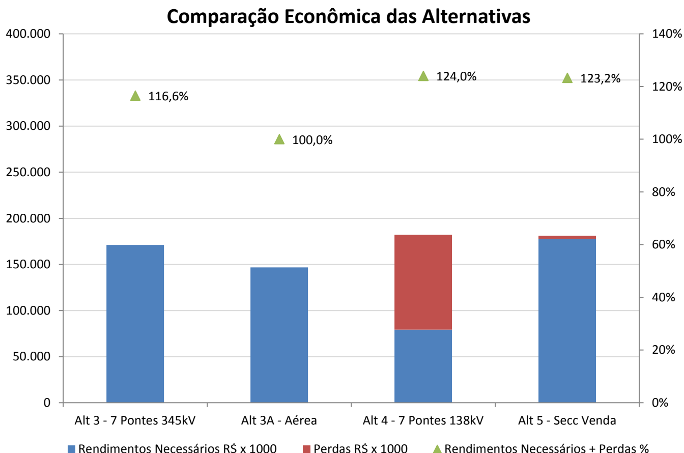
Figura 10-2 - Gráfico de comparação econômica de alternativas
