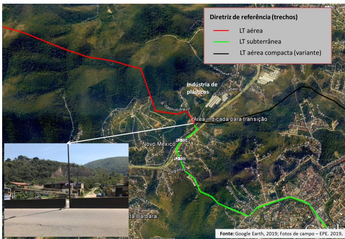
Figura 10 – Indicação de possível área para a segunda estação de transição LT aérea / LT subterrânea
