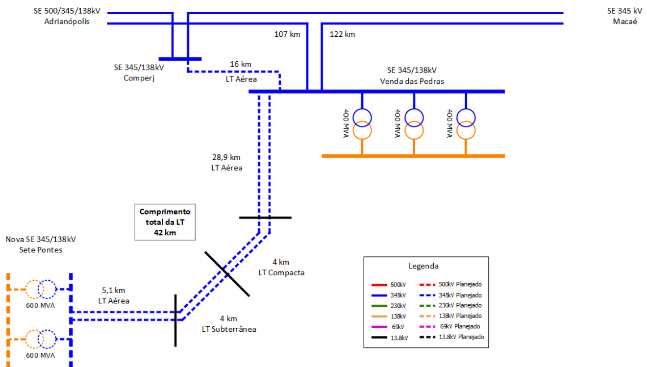
Figura 3-1 - Representação simplificada da alternativa 3
