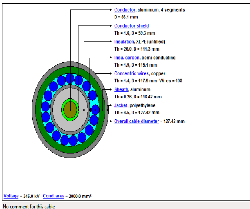
Figura 9-4 Dados construtivos do cabo de alumínio 2000 mm² de 345 kV
