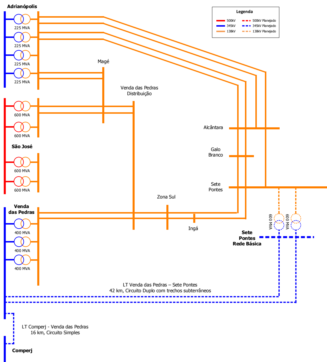
Figura 6-5 - Diagrama simplificado das principais obras da Alternativa 3
